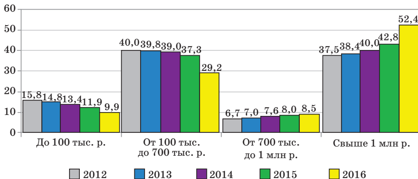
Рис. 2. Структура депозитов в зависимости от размера вкладов в 2012–2016 гг. (на 1 января), %
